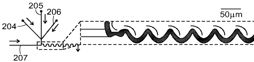
FIG. 2B-2
