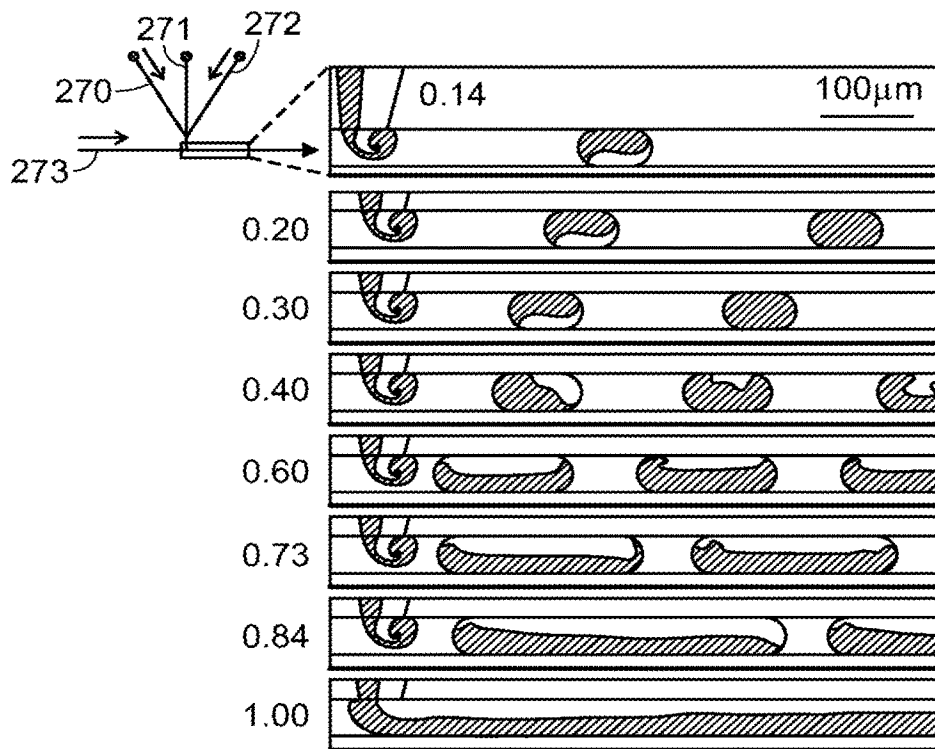
FIG. 27B
