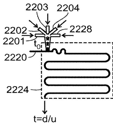
FIG. 22A
