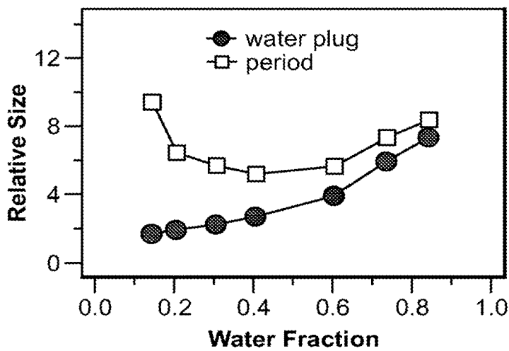
FIG. 29B
