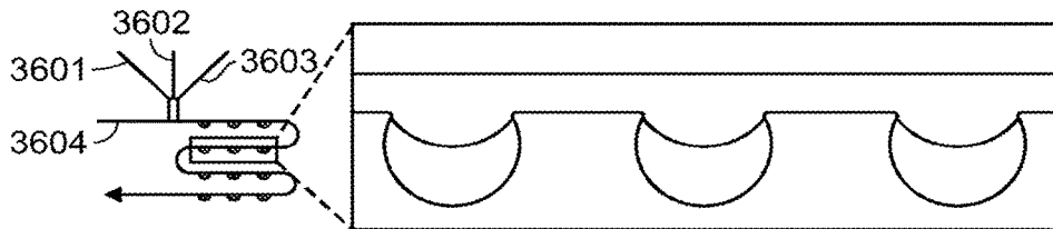
FIG. 36
