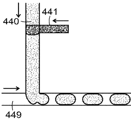
FIG. 44A
