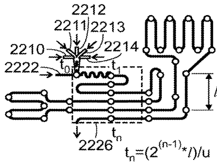
FIG. 22C
